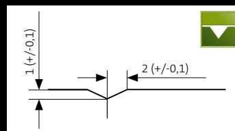
2V – chanfrein standard
