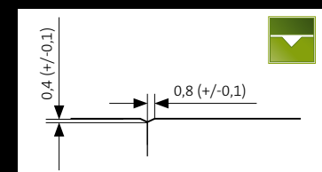
2mV – Mikrofase
