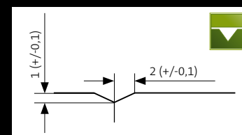
2V – Standardfase
