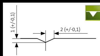
2V – стандартная фаска
