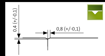
2mV – micro bisellatura
